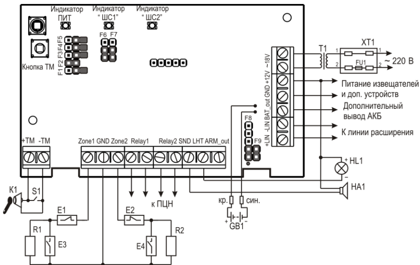
Рисунок А.2- Схема подключения извещателей, имеющих выход типа «сухой контакт» (релейный), и работающих на замыкание или размыкание
