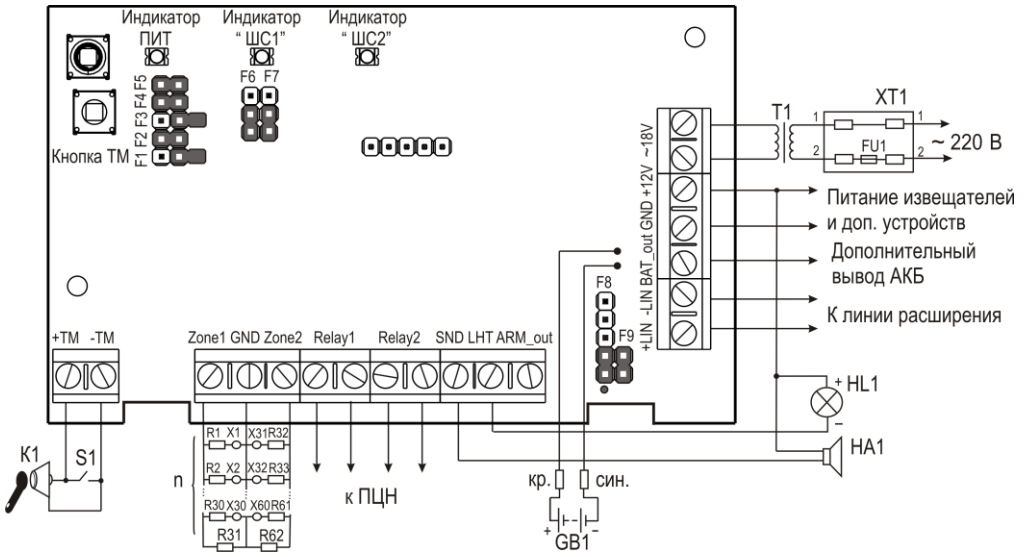
Рисунок А.3- Схема подключения активных извещателей
